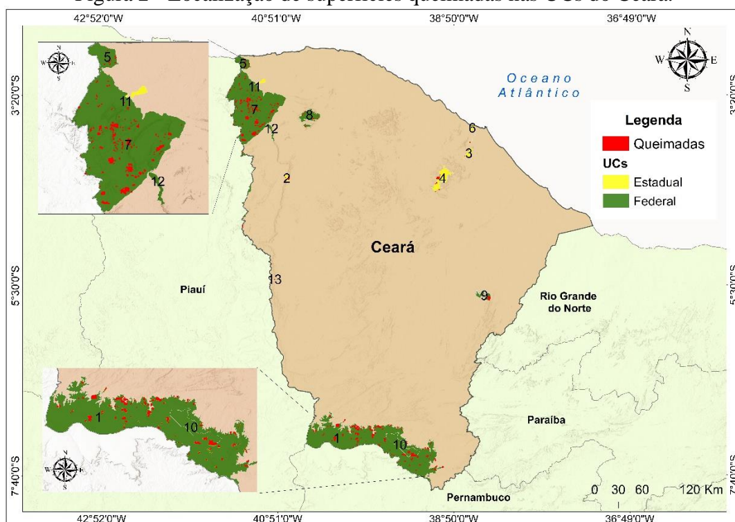
Figura 2 - Localização de superfícies queimadas nas UCs do Ceará.
