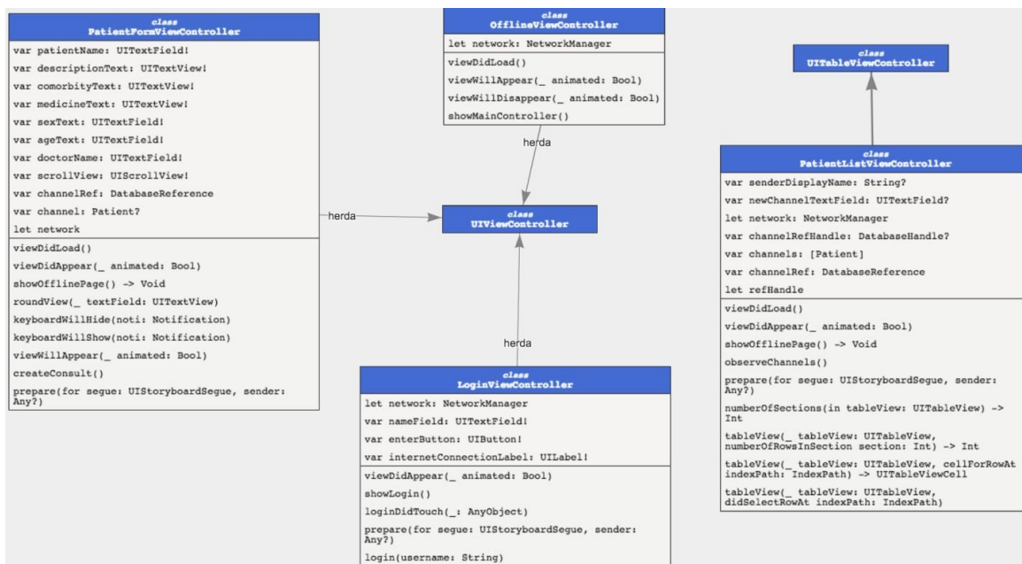
FIGURA 4 - Diagrama de classes do aplicativo Ceanne Hospital
