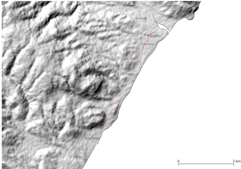
Figura S1: DEM sin procesar, representado como relieve sombreado. Nótese los píxeles sin datos, destacados en color rojo (Los Patos-Ojeda-Paraíso, provincia Barahona, sudoeste de República Dominicana)
