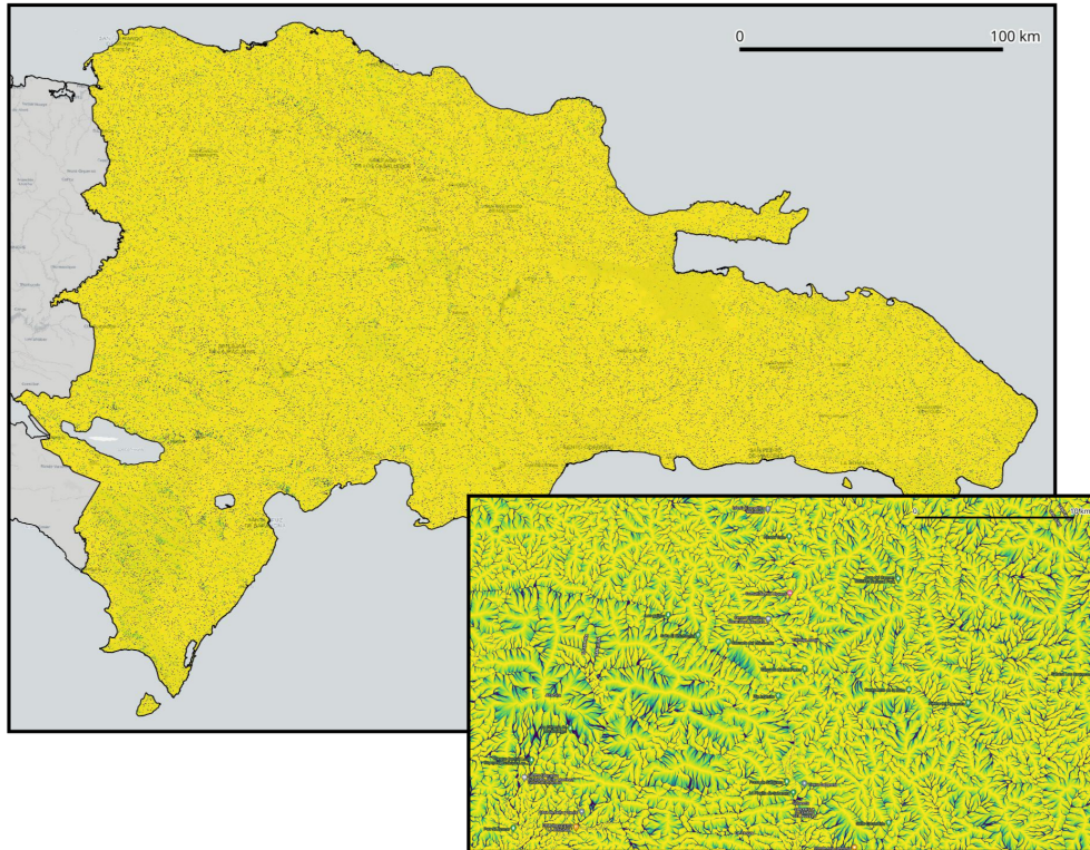
Figura S9: Mapa de acumulación de flujo generado con 'r.watershed'. En cartela, detalle del mapa en la cuenca del río Yaque del Sur.
