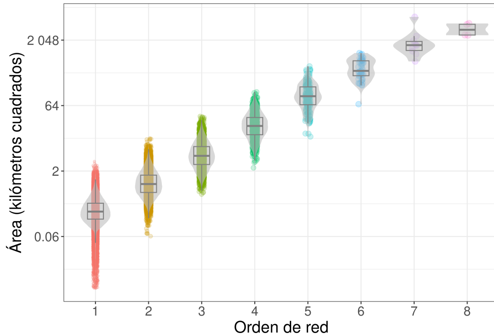
Figura 6: Área de las cuencas y subcuencas según órdenes de red de Strahler para el umbral de acumulación 540 celdas ( \sim 8 hectáreas)
