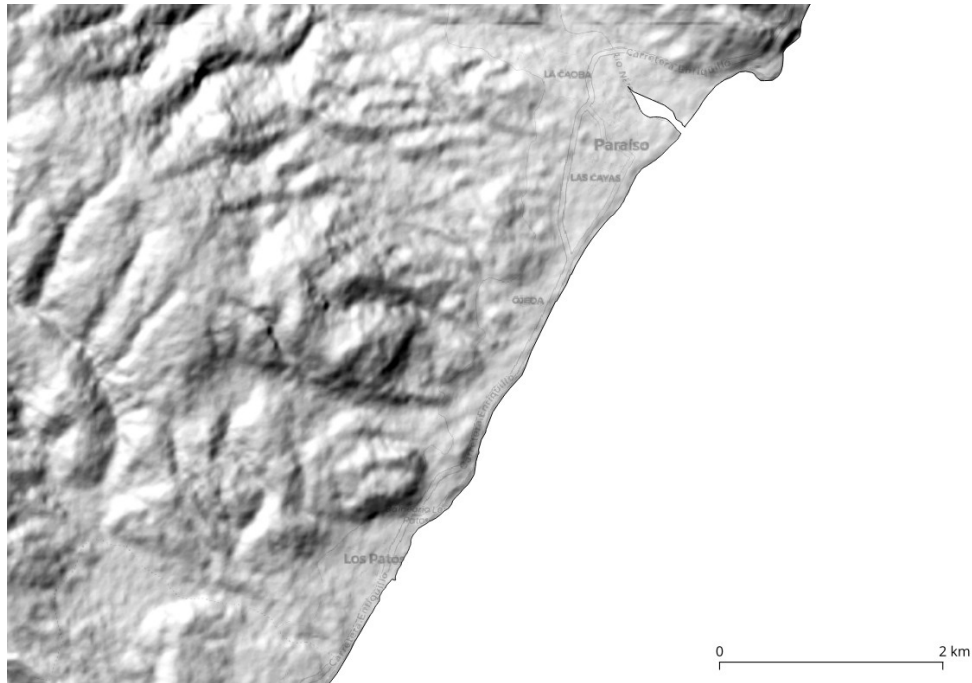
Figura S2: DEM sin procesar, representado como relieve sombreado. Los píxeles sin datos fueron eliminados (Los Patos-Ojeda-Paraiso, provincia Barahona, sudoeste de República Dominicana)
