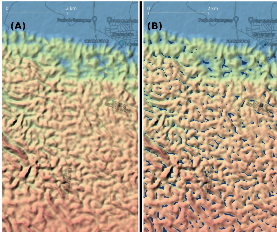
Figura S8: DEM ALOS PALSAR representado como mapa hipsométrico (rojo y marrón representan terreno elevado, verde y azul claro terreno bajo) sobre relieve sombreado, mostrando el área de Guaraguaio, Los Haitises, al sur del río Yuna (nordeste de República Dominicana). (A) sin mostrar depresiones, (B) mostrando depresiones en tonalidad azul oscuro
