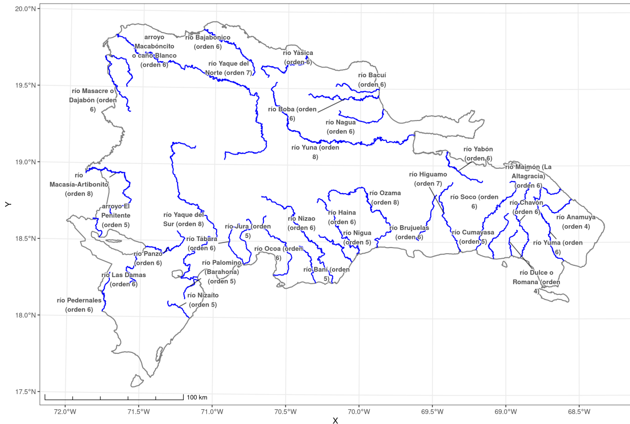
Figura 10: Cursos más largos de 35 ríos seleccionados de la República Dominicana basados en orden de red y representatividad territorial. Se priorizaron ríos de orden seis o superior. En áreas del sur y sudoeste, se incluyeron ríos de orden cinco de notable longitud.
