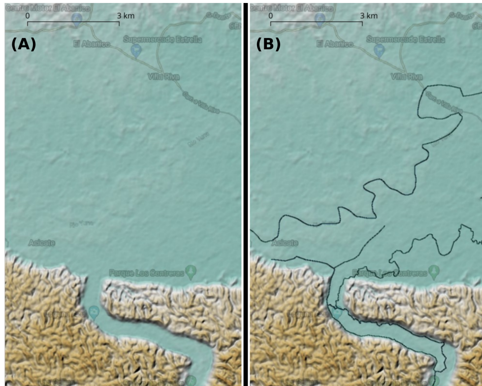
Figura S6: DEM sin aplicación de hidrografía (A), y con aplicación de hidrografía seleccionada o "DEM tallado"(B). El DEM se representa como relieve sombreado y la aplicación se denota como un grabado oscurecido (cañón del río Payabo, Los Haitises, y río Yuna (proximidades de Arenoso, nordeste de República Dominicana)
