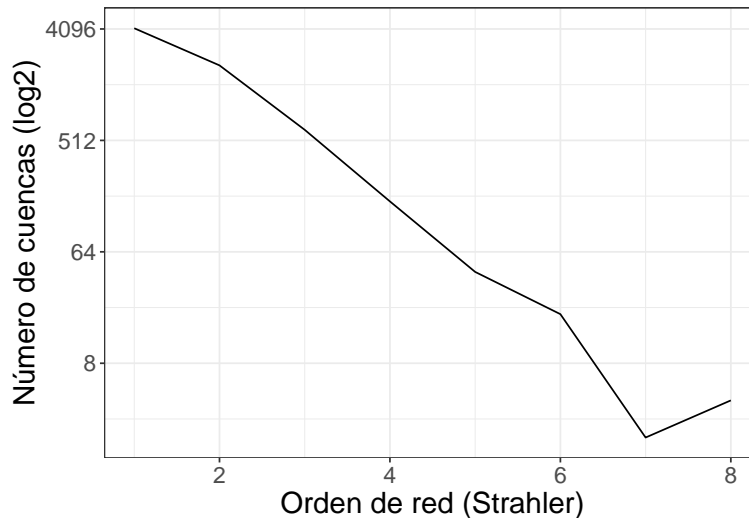
Figura 5: Número de cuencas que desembocan en mares, lagos, lagunas o en pérdidas kársticas, según órdenes de red de Strahler para el umbral de acumulación 540 celdas ( \sim 8 hectáreas)
