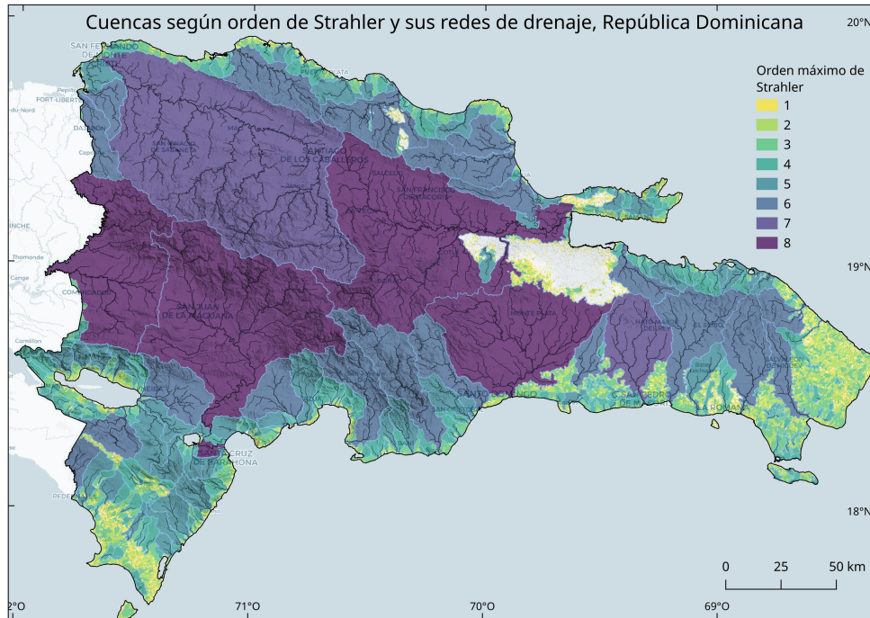
Figura 4: Cuencas que desembocan en mares, lagos, lagunas o en pérdidas kársticas categorizadas según orden de Strahler de República Dominicana, y sus correspondientes redes de drenaje (sólo mostrando los cursos de orden 4 o superior). El umbral de acumulación usado para extraer la red fue de 540 celdas (aprox. 8 ha).
