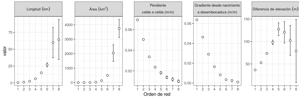
Figura 9: Promedios de longitud de cursos, área de cuenca, pendiente (celda a celda), gradiente (entre extremos) y rango promedio (diferencia de elevación), por tramos, según órdenes de Strahler
