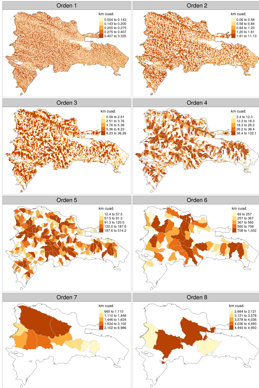
Figura 7: Distribución espacial de las cuencas y subcuencas según superficie calculada y órdenes de red de Strahler para el umbral de acumulación 540 celdas (~8 hectáreas)
