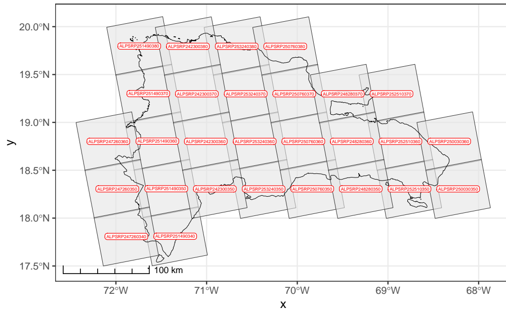
Figura 2: Mapa índice de las 28 escenas usadas en la formación del DEM de República Dominicana, superponiendo las huellas (polígono de área con datos) de las escenas ALOS PALSAR RTC sobre el límite costero e internacional del país
