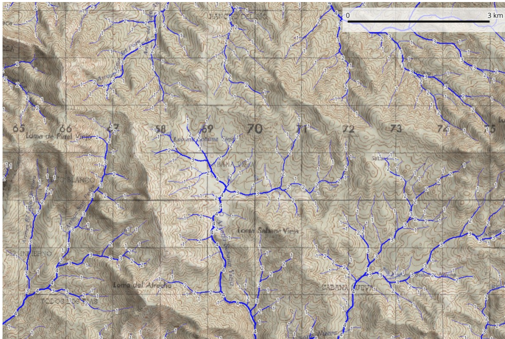
Figura S12: Orden de red de Strahler en el área del pico de la Viuda y Sabana Vieja, provincia San Juan (vertiente sur de la cordillera Central de República Dominicana). Esta red fue generada usando un umbral de acumulación de 180 celdas, equivalente a 3 ha. De fondo, mapa topográfico nacional escala 1:50,000 y relieve sombreado
