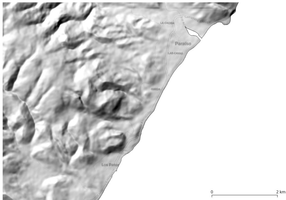
Figura S3: DEM suavizado, representado como relieve sombreado. Nótese la conservación de las morfologías principales y la eliminación del ruido sobre éstas (Los Patos-Ojeda-Paraiso, provincia Barahona, sudoeste de República Dominicana)
