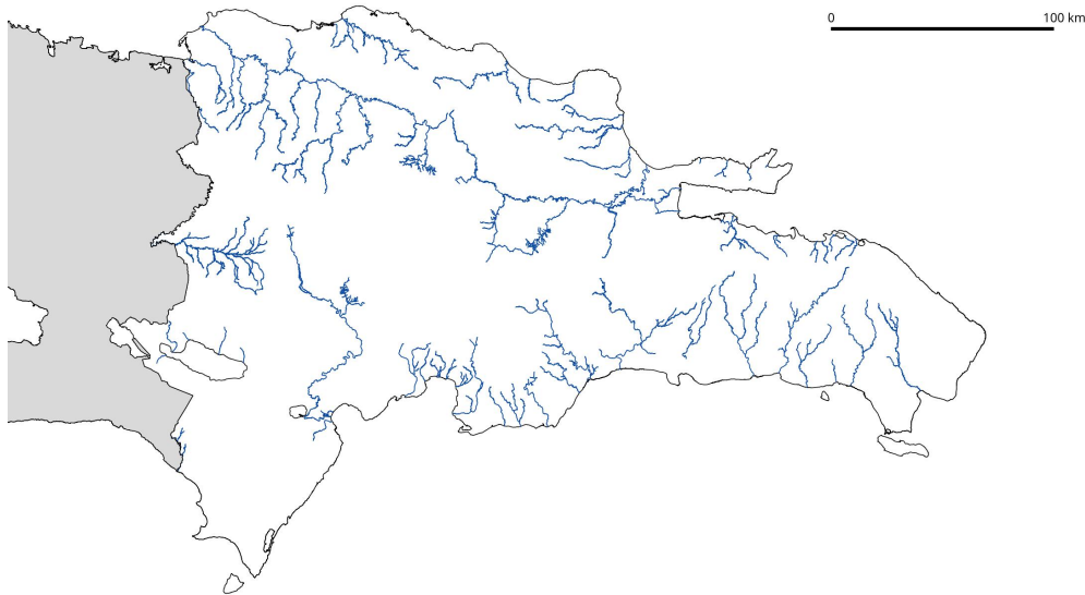
Figura S5: Mapa de la red de cursos largos creada para el estudio a partir de varias fuentes (más detalles, en el texto).
