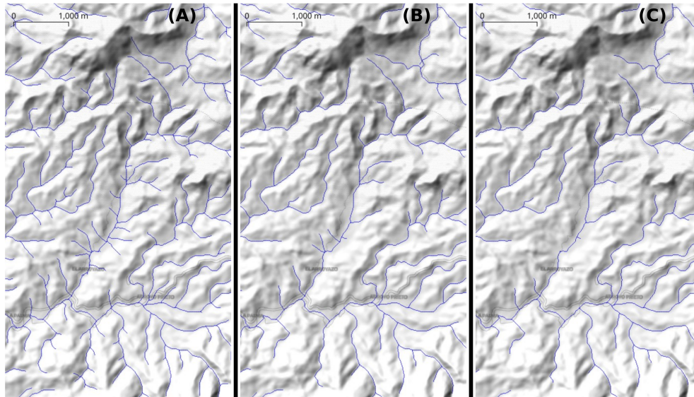
Figura S10: Red de drenaje extraída para tres umbrales de acumulación: (A) 180 celdas, equivalente a 3 ha; (B) 540 celdas, equivalente a 8 ha; (C) 900 celdas, equivalente a 14 ha. La imagen de fondo es un relieve sombreado a partir de DEM ALOS PALSAR, mostrando el área de El Arroyazo en la reserva científica Ébano Verde (provincia La Vega, cordillera Central de República Dominicana)
