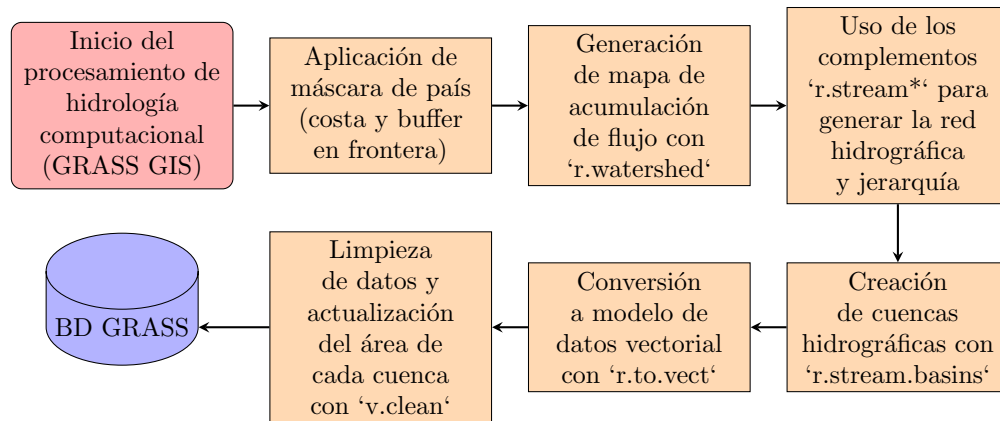
Figura 3: Resumen gráfico del procesamiento de hidrología computacional
