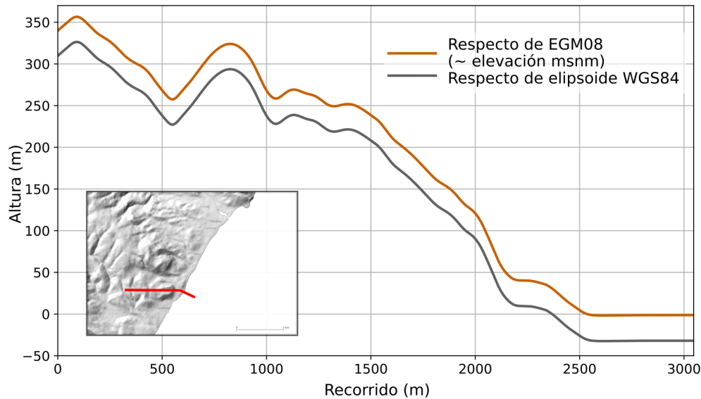
Figura S4: Alturas respecto de geoide EGM08 (~ortométrica) y sobre elipsoide WGS84, de un transecto descendente desde Bahoruco Oriental al Mar Caribe (Los Patos-Ojeda-Paraíso, provincia Barahona, sudoeste de República Dominicana)
