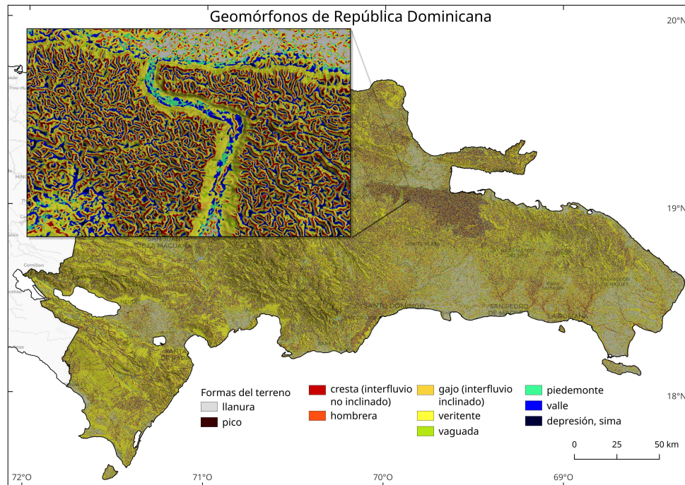
Figura S7: "Geomórfonos" de República Dominicana generados a partir de DEM ALOS PALSAR. En cartela, detalle del cañón del río Payabo
