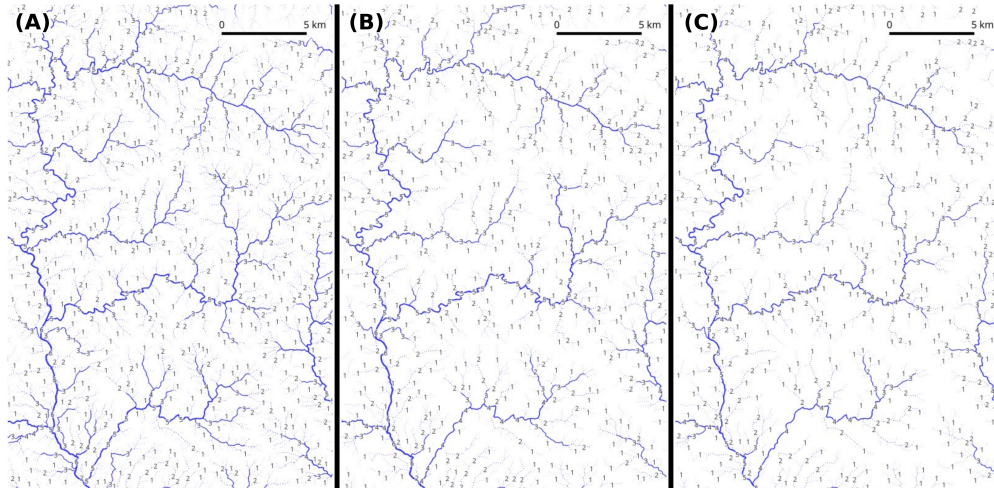
Figura S11: Orden de red de Strahler para redes de drenaje generadas a partir de tres umbrales de acumulación: (A) 180 celdas, equivalente a 3 ha; (B) 540 celdas, equivalente a 8 ha; (C) 900 celdas, equivalente a 14 ha. El área mostrada corresponde al río San Juan, afluente del río Yaque del Sur (vertiente sur de la cordillera Central de República Dominicana)
