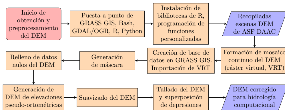
Figura 1: Resumen gráfico de la obtención y preprocesamiento del DEM
