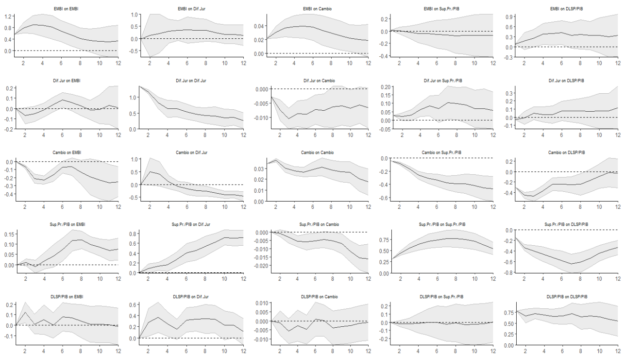
Figura 2 Função impulso resposta a partir de Projeções Locais (Lineares). Dados mensais, jan. 1999 a nov. 2022 10
