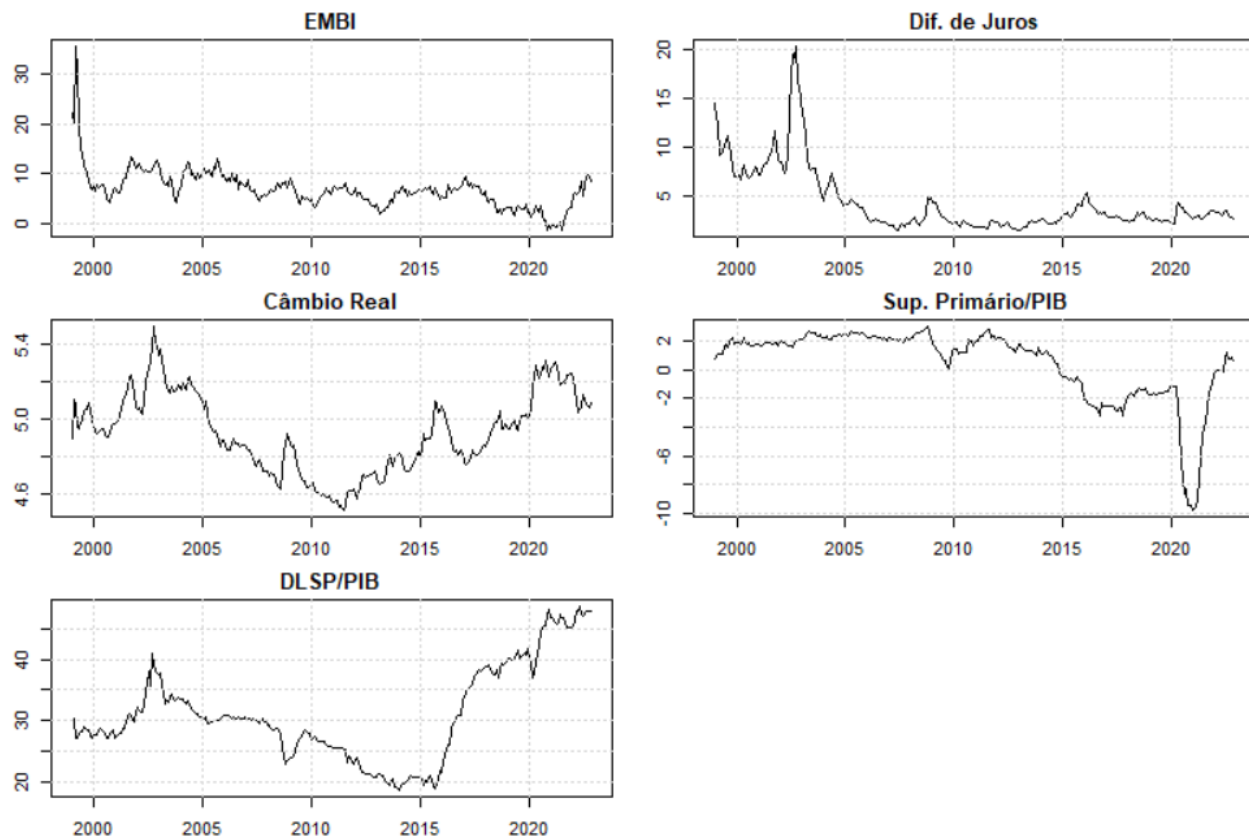
Figura 1 Comportamento das variáveis utilizadas nas estimativas econométricas. Dados mensais, jan. 1999 a nov. 2022.
