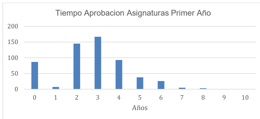
Figura 4. Histograma Tiempo Aprobación Asignaturas Año 1
