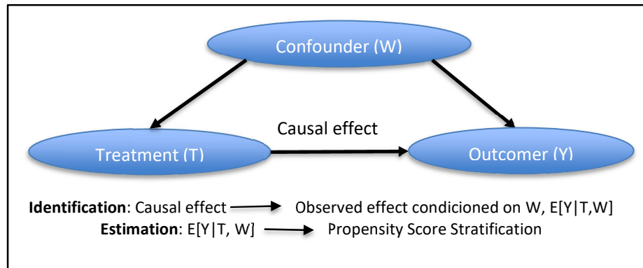
Figura 2. Grafo de relación causal (DAG)
