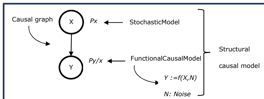
Figura 1. Estructura del Modelo Causal
