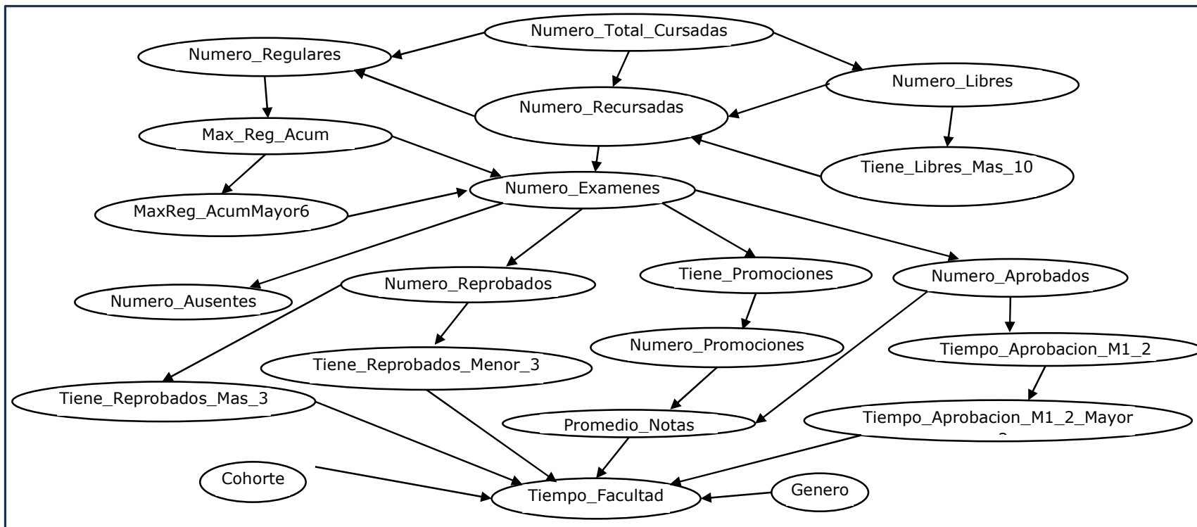
Figura 5. Grafo Causal Directo Acíclico (DAG)
