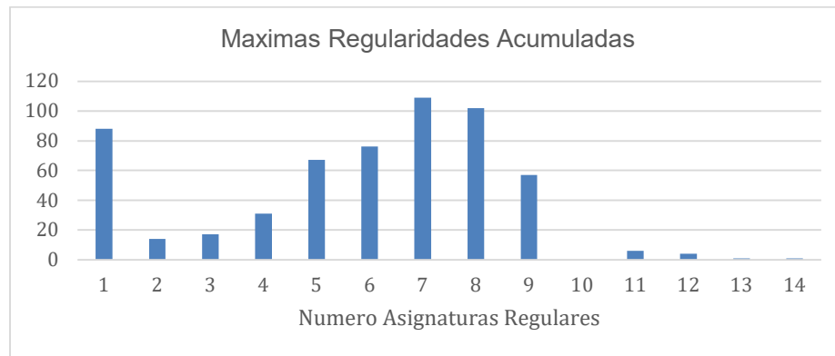
Figura 3. Histograma Máximas Regularidades Acumuladas
