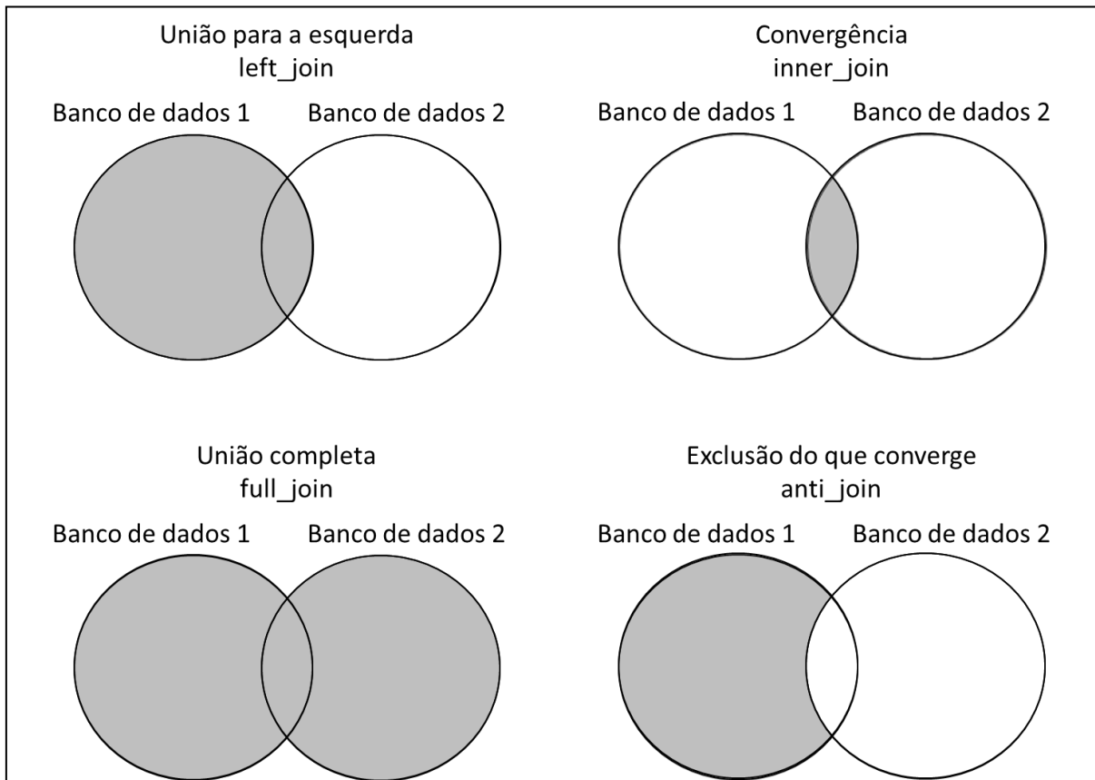
Figura 1 – Representação dos tipos de união de banco de dados, segundo funções do software R
