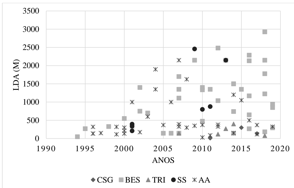
Figura 3 Evolução das capacidades operacionais em profundidade de LDA por subsistemas de processamento submarino (1990-2019)
