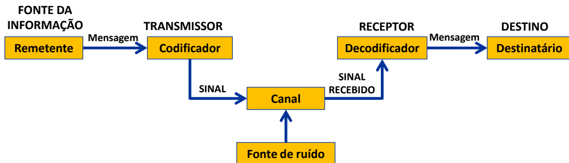
Figura 1: Modelo de Comunicação Centrado na Informação
