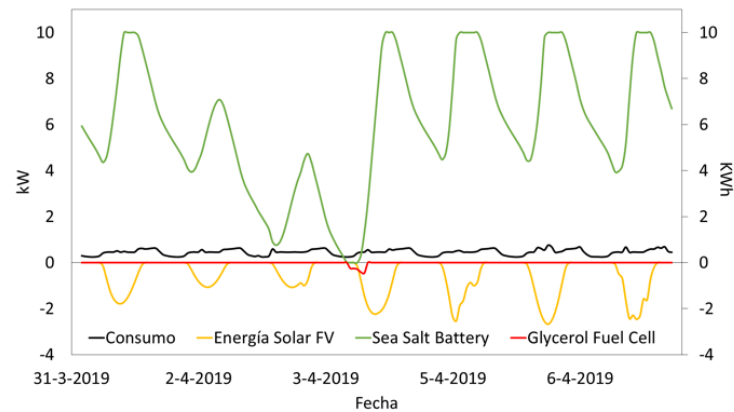
Figura 3. Resultados de BEopt y DstorageS de consumo de una vivienda con electricidad neutral en Colombia con energía solar FV, una batería de sal marina y una celda de combustible de glicerol durante la primera semana de abril 2019.
