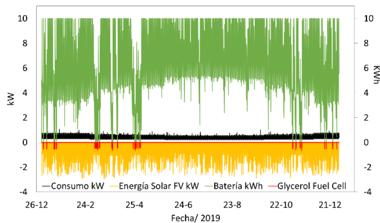
Figura 5. Resultados de BEopt y DstorageS de consumo de una vivienda con electricidad neutral en Colombia con energía solar FV, una batería de sal marina y una celda de combustible de glicerol durante el año 2019.
