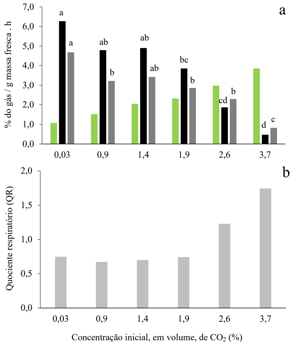
Figura 2. Porcentagem de CO 2 registrada no frasco de 600 mL (a, barras verdes), consumo de O 2 (a, barras pretas) e liberação de CO 2 (a, barras cinzas) registrados nesse mesmo frasco e quociente respiratório (b) das sementes de Eugenia brasiliensis Lam. incubadas a 25 °C por 17 horas em atmosferas com diferentes concentrações de CO 2 . Médias seguidas da mesma letra não diferem estatisticamente, de acordo com o teste de Tukey ao nível de 5%.
