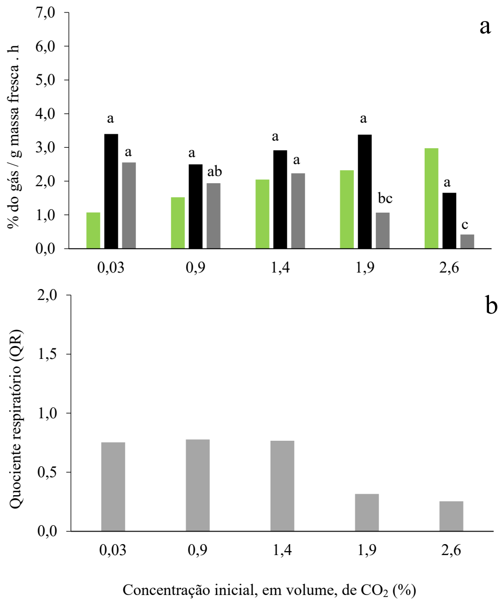
Figura 3. Porcentagem de CO 2 registrada no frasco de 600 mL (a, barras verdes), consumo de O 2 (a, barras pretas) e liberação de CO 2 (a, barras cinzas) registrados nesse mesmo frasco e quociente respiratório (b) das sementes de Eugenia brasiliensis Lam. incubadas a 25 °C por 41 horas em atmosferas com diferentes concentrações de CO 2 . Médias seguidas da mesma letra não diferem estatisticamente, de acordo com o teste de Tukey ao nível de 5%.
