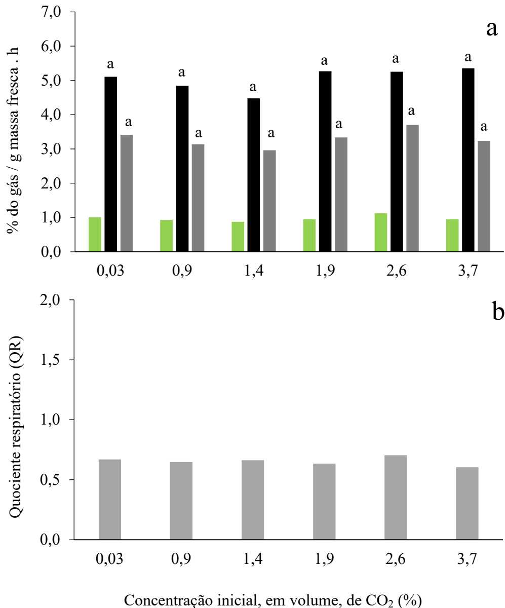
Figura 4. Porcentagem de CO 2 registrada no frasco de 600 mL (a, barras verdes), consumo de O 2 (a, barras pretas) e liberação de CO 2 (a, barras cinzas) registrados nesse mesmo frasco e quociente respiratório (b) das sementes de Eugenia brasiliensis Lam. incubadas a 25 °C por 24 horas após reabertura dos frascos para normalizar a atmosfera. Médias seguidas da mesma letra não diferem estatisticamente, de acordo com o teste de Tukey ao nível de 5%.
