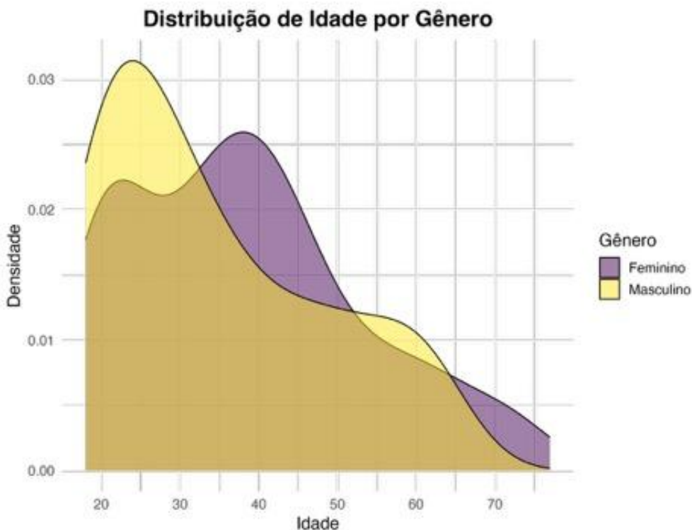
Gráfico 3. Distribuição de idade dos participantes segundo o gênero (feminino, masculino). As curvas representam a densidade estimada da distribuição de idade em cada grupo.
